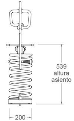
vista lateral 1:20
