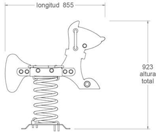
vista alzado 1:20
