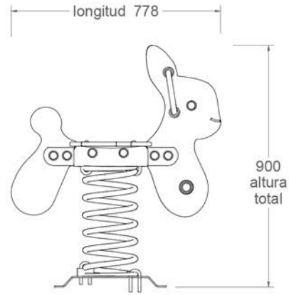
vista alzado 1:20
