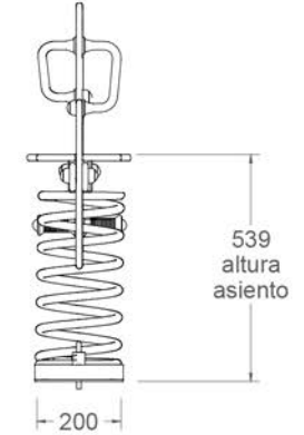
vista lateral 1:20
