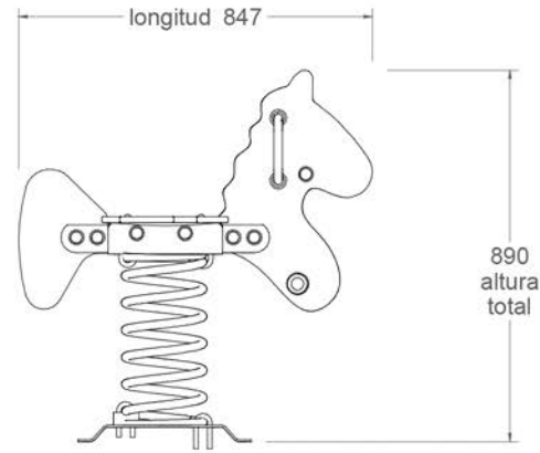
vista alzado 1:20
