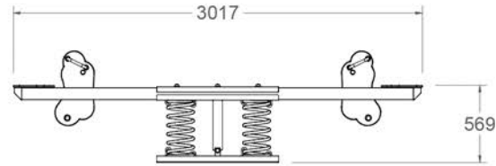
vista alzado 1:50
