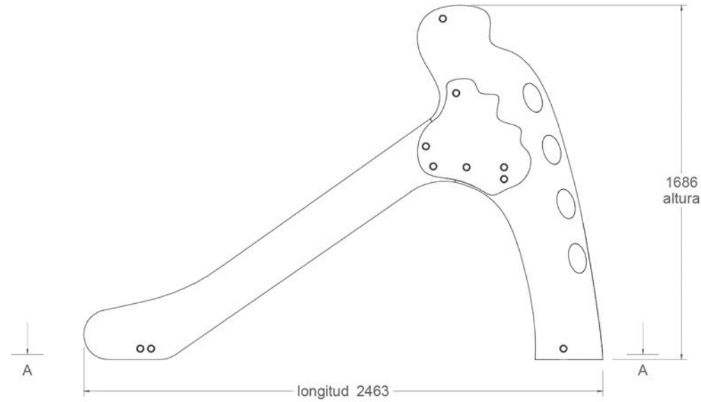
vista alzado 1:25
