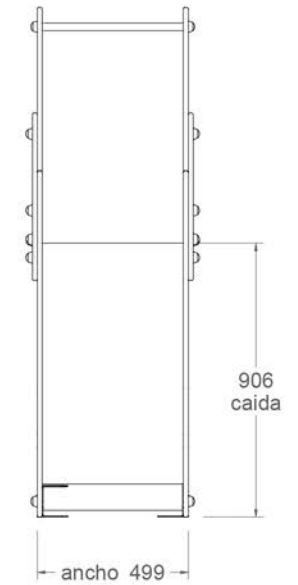
vista lateral 1:25
