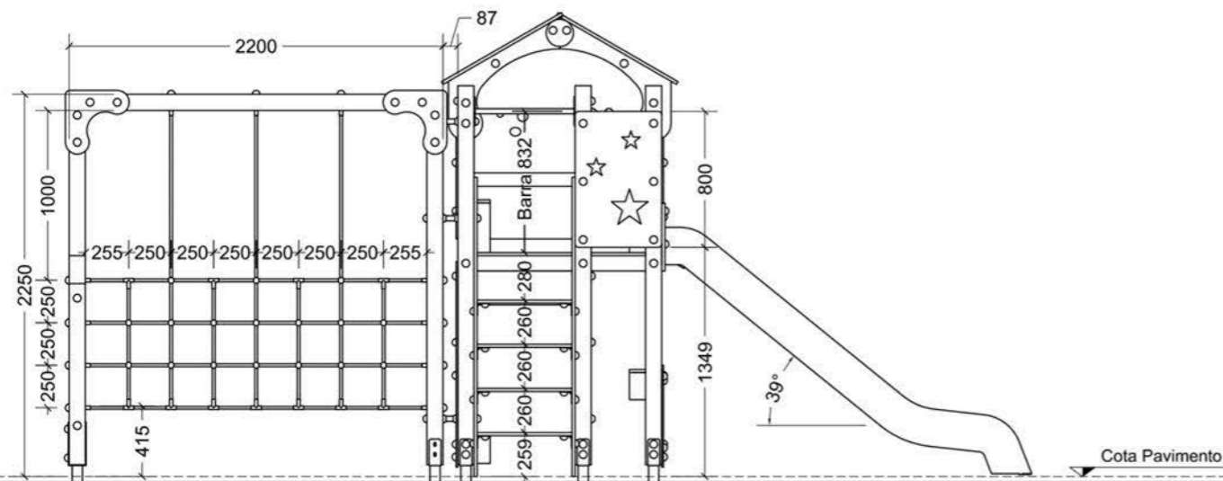
Alzado Frontal
