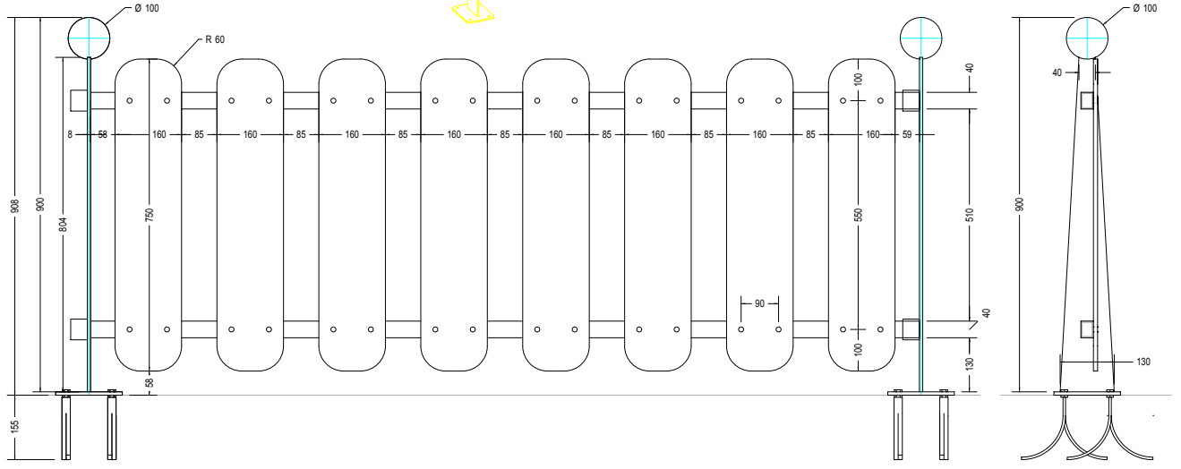
Alzado
