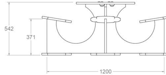
vista alzado 1:20
